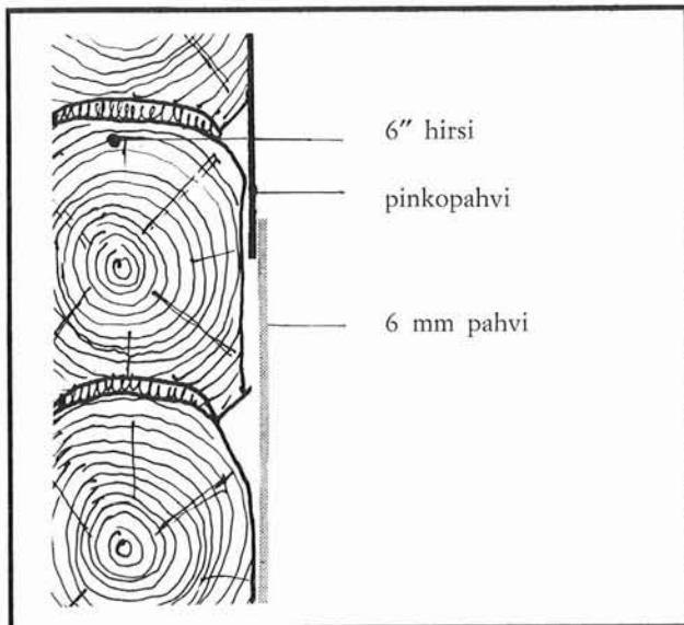
Hoitohuoneiden sisäisten seinien yleisin rakenne: 6" hirren päälle kiinnitettyä 6 mm paksuinen pahvi, jollainen ulottui lattiapinnasta 140 cm korkeuteen, josta ylöspäin verhouksena oli pinkopahvi. Henkilökunnan asunnoissa oli pabvien päällä lisäksi useita tapettikerroksia sekä huokoinen puukuitulevy. Samanlainen seinärakenne on yleinen kunnalliskodin muillakin osastoilla.
