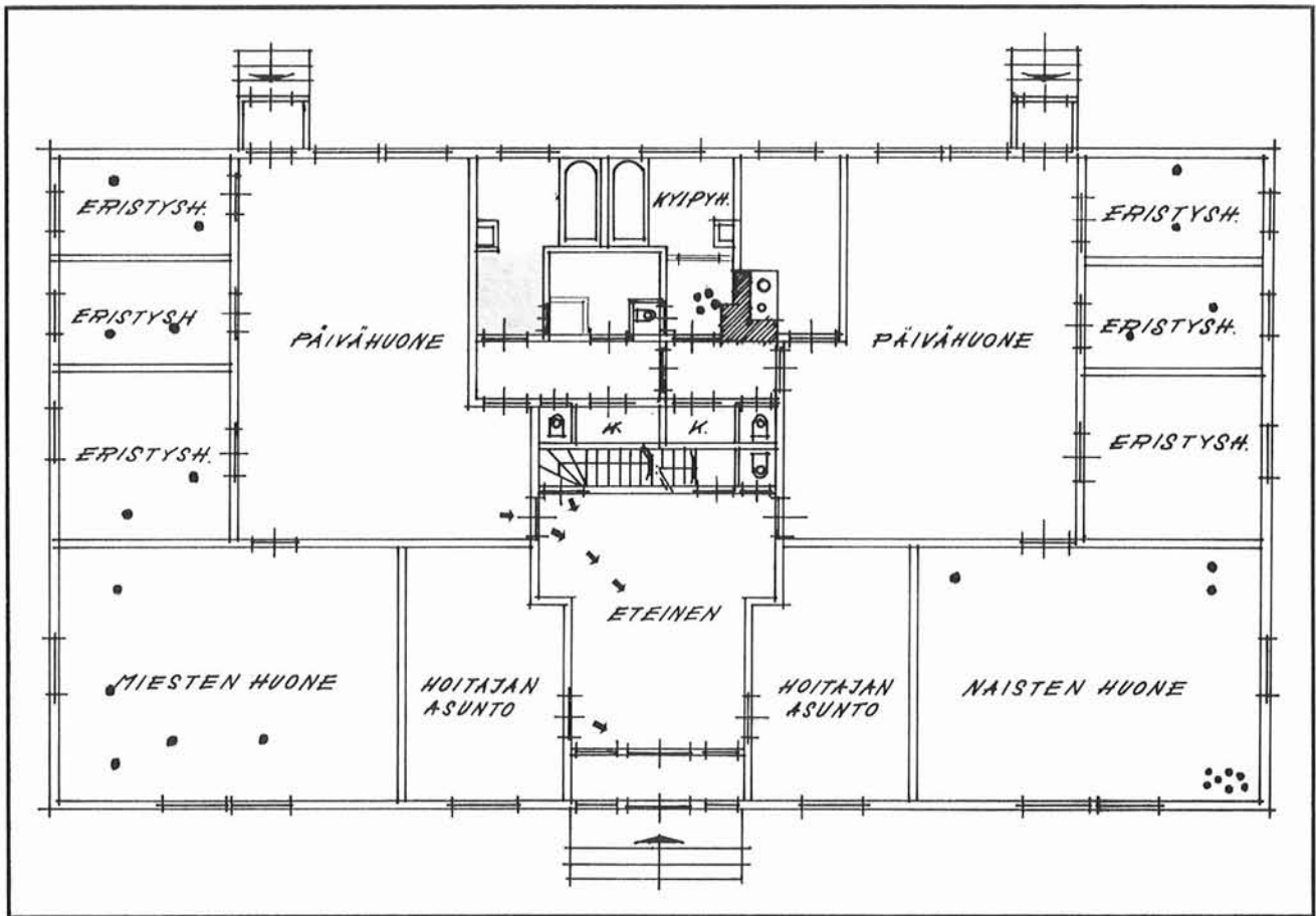
Mielisairasosaston hoitokerros. Keskiosassa varjostettuna miesten tupakkahuoneesta alue, josta palon on todettu saaneen alkunsa ja levinneen ensin ovien kautta miesten päivähuoneeseen ja sieltä avatun oven kautta eteishalliin ja edelleen naisten osastolle sinne johtaneen lukitun oven yläpuolisesta ikkunasta. Kuvaa on merkitty nuolin pelastuneiden pakotiet ja mustin pistein ruumiiden löytöpaikat. Varauksikäytävät piirroksen yläosassa.
